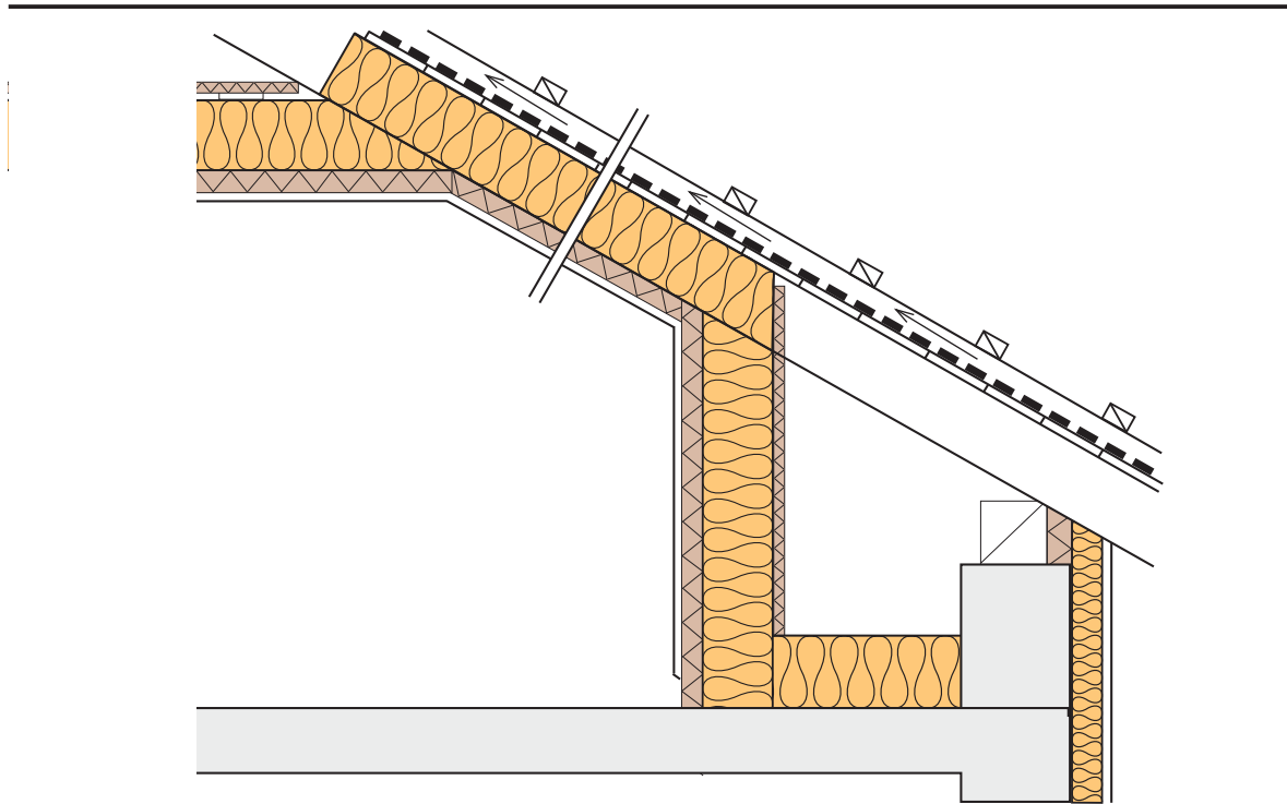
Рисунок 3. Схема устройства теплового контура скатной кровли
