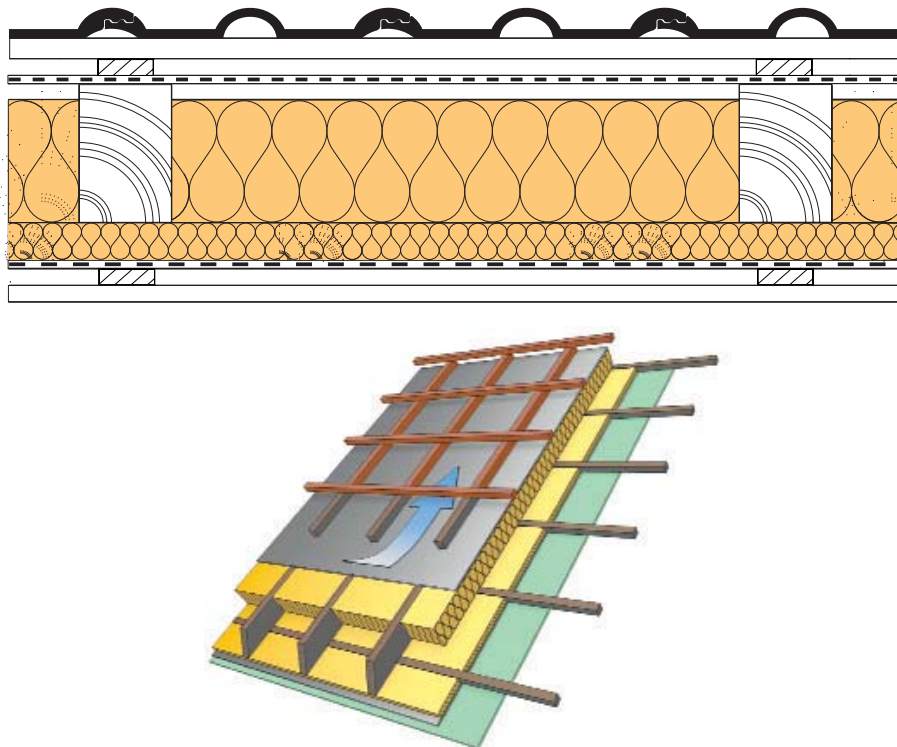
Рисунок 8. Устройство дополнительного слоя теплоизоляции с внутренней стороны
