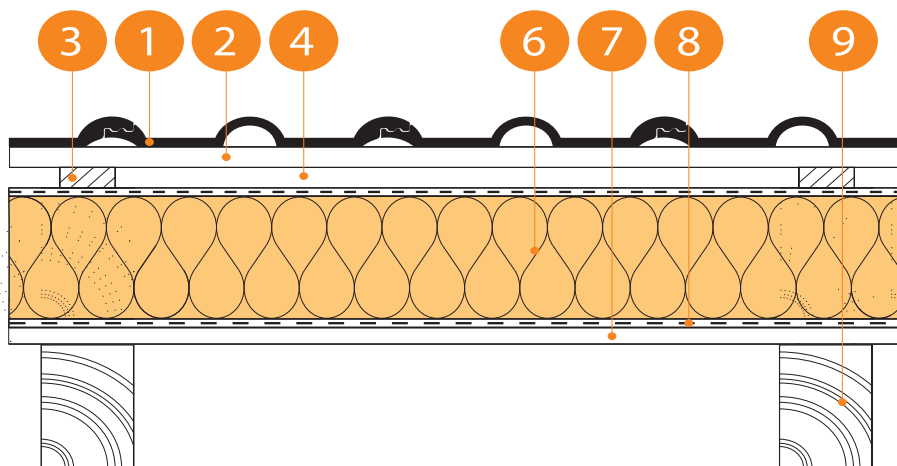
Рисунок 5. Кровля с размещением слоя теплоизоляции с наружной стороны стропильной конструкции, Вариант 2
