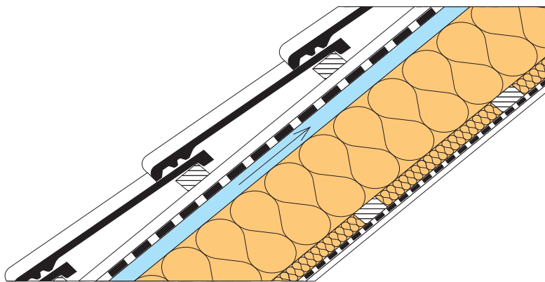
Рисунок 2. Утепление скатной кровли с организацией воздушного зазора
