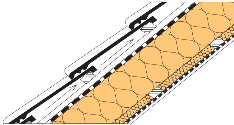
Рисунок 1. Утепление скатной кровли традиционным методом без воздушного зазора
