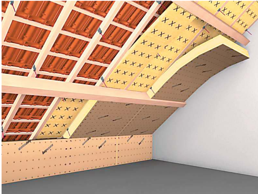
Рисунок 6. Утепление кровли со стороны внутреннего объема подстропильного пространства
