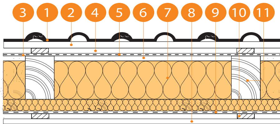
Рисунок 7. Кровля с организацией дополнительного воздушного зазора, Вариант 3
