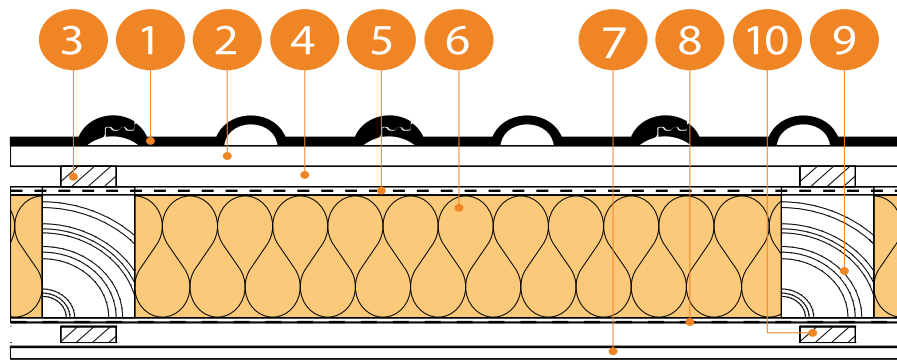
Рисунок 4. Кровли с размещением слоя теплоизоляции в межстропильном пространстве, Вариант 1
